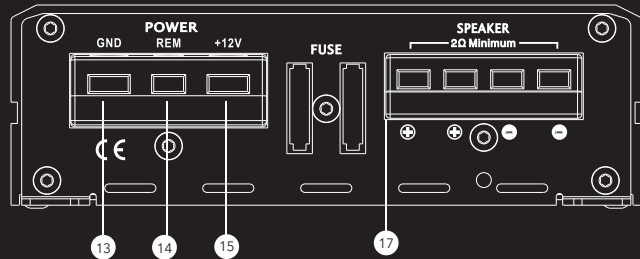
MPD 1.500 - Back panel
